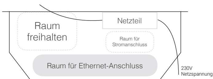
Unterputz-Hohlwanddose, Schnittansicht (Längsseite)
